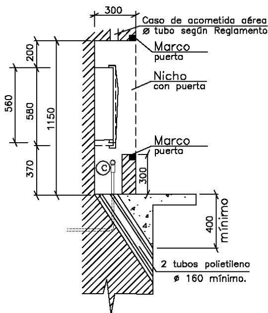
SECCION A-A'
