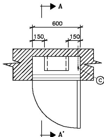
PLANTA
