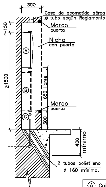
SECCION A-A'
